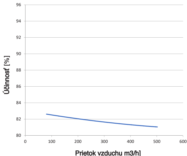
Výkonová krivka HRU-PremAIR-500
