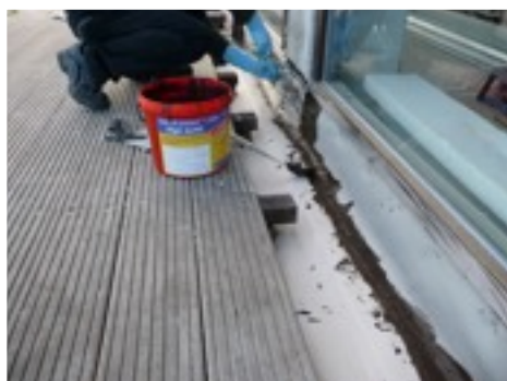
Aplikácia náter detail dvere
