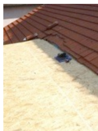
Aplikacia na drevo +špec.membrána,TG
